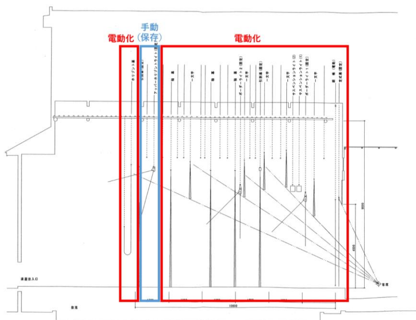
【舞台断面図】
