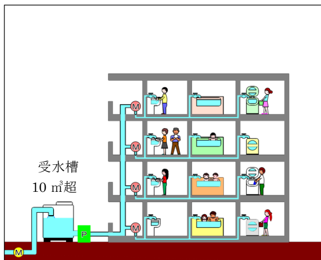
受水槽加圧ポンプ方式の場合
