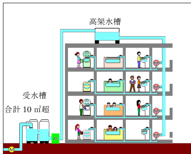
高架水槽方式の場合(受水槽合計 10 m 3 を超えるもの)
