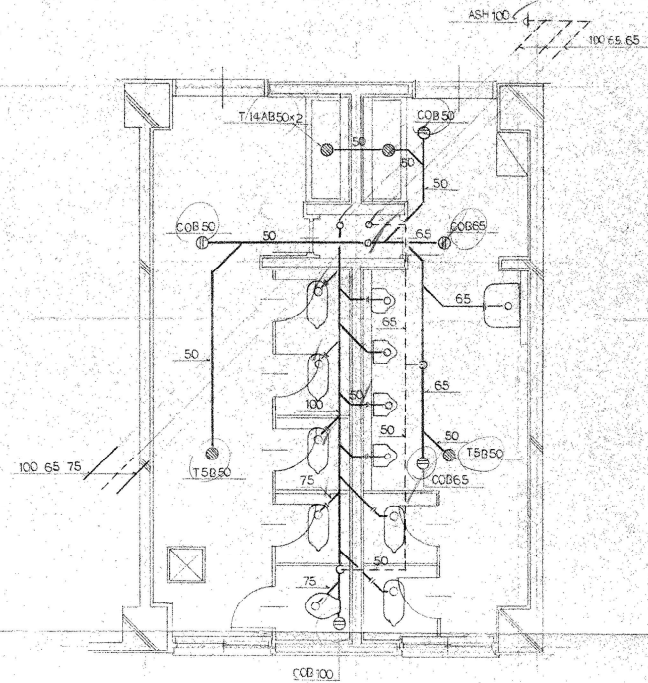
2階生徒使用 1/50
