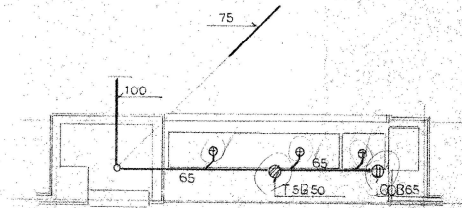
1階廊下流し S 1/50
