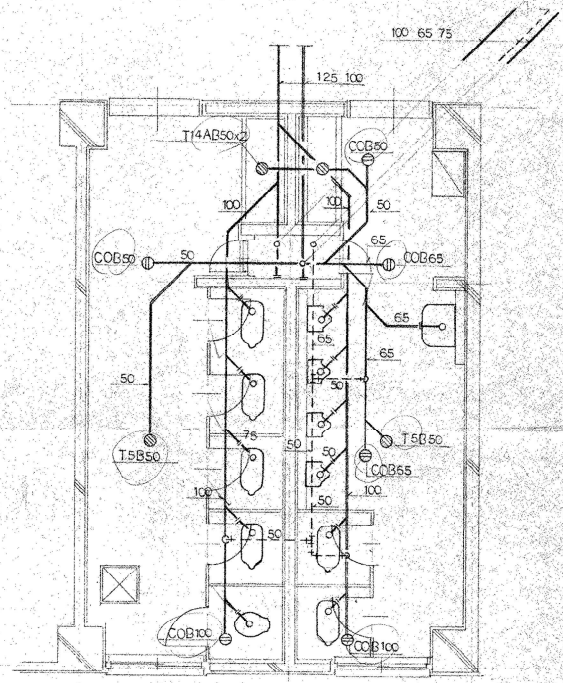
1階生徒便所 S 1/50
